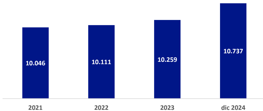
Capacidad de Transformación [MVA]
